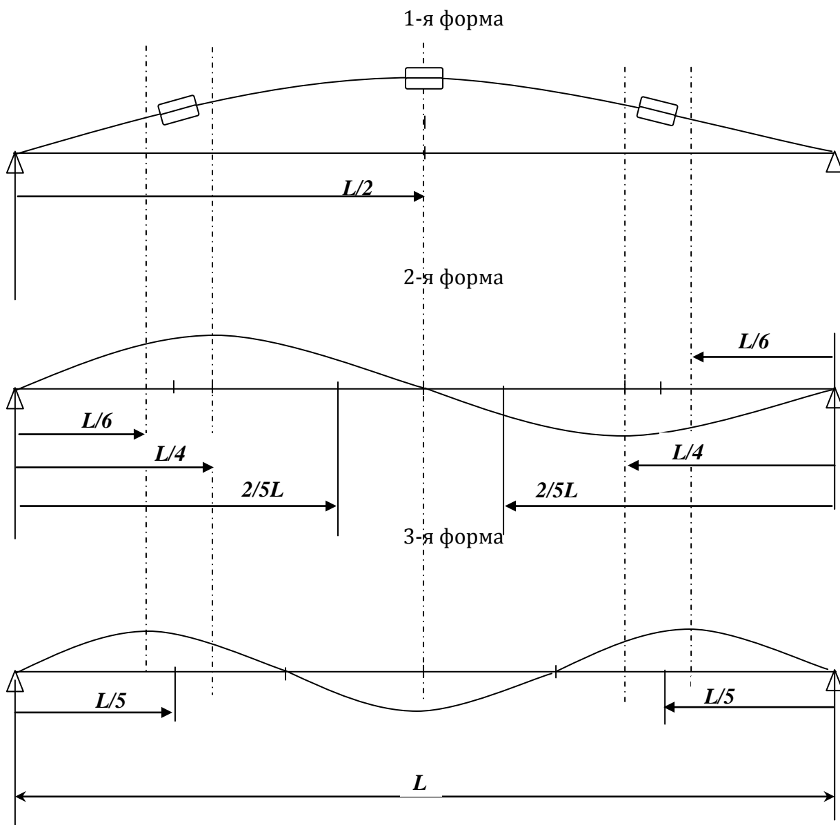
Рис. 4. Схемы расстановки гасителей ГВКУ
